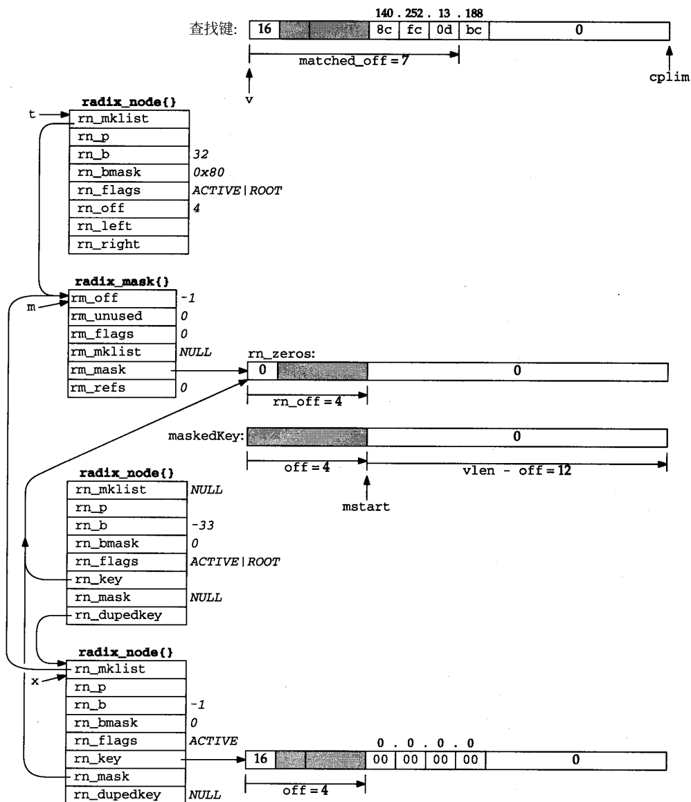
图18-47 回溯到路由树的顶端和查找默认叶子的 rn_search
