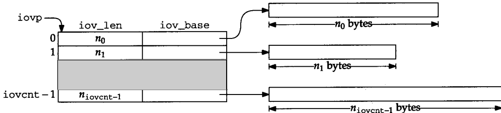
图16-11 writerv 系统调用中的 iovec 参数
