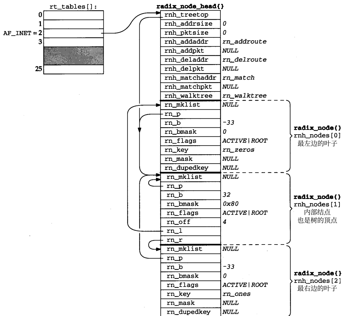
图18-34 rn_inithead 为Internet协议创建的 radix_node_head 结构
