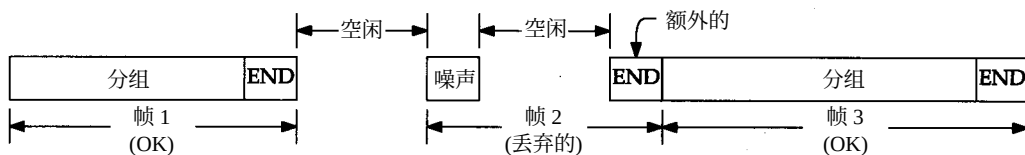
图5-18 Karn的丢弃SLIP线路噪声的方法
