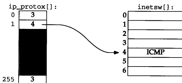
图11-13 数值为1的ip_p 选择了 inetsw[4]
