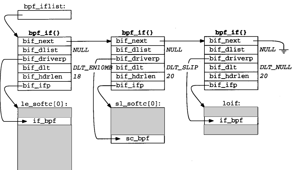
图31-7 bpf_if 和ifnet 结构
