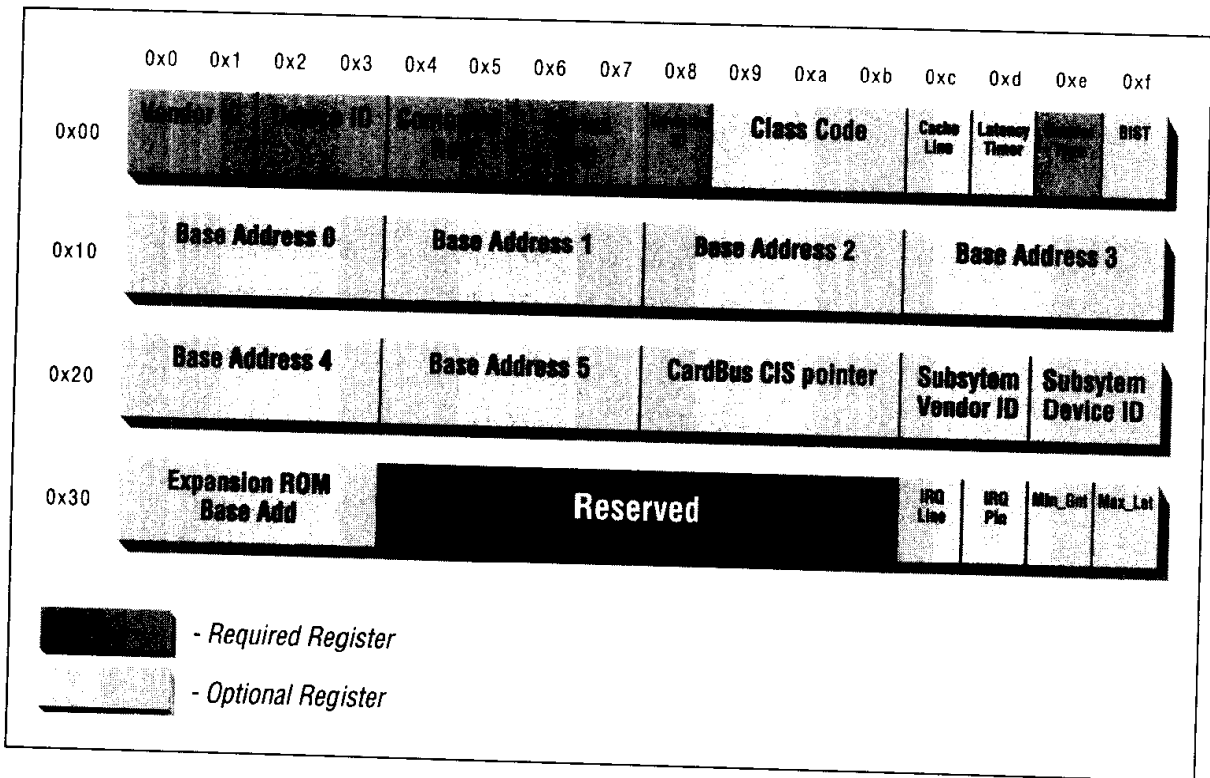
图 15-1 标准化的 PCI 配置寄存器
