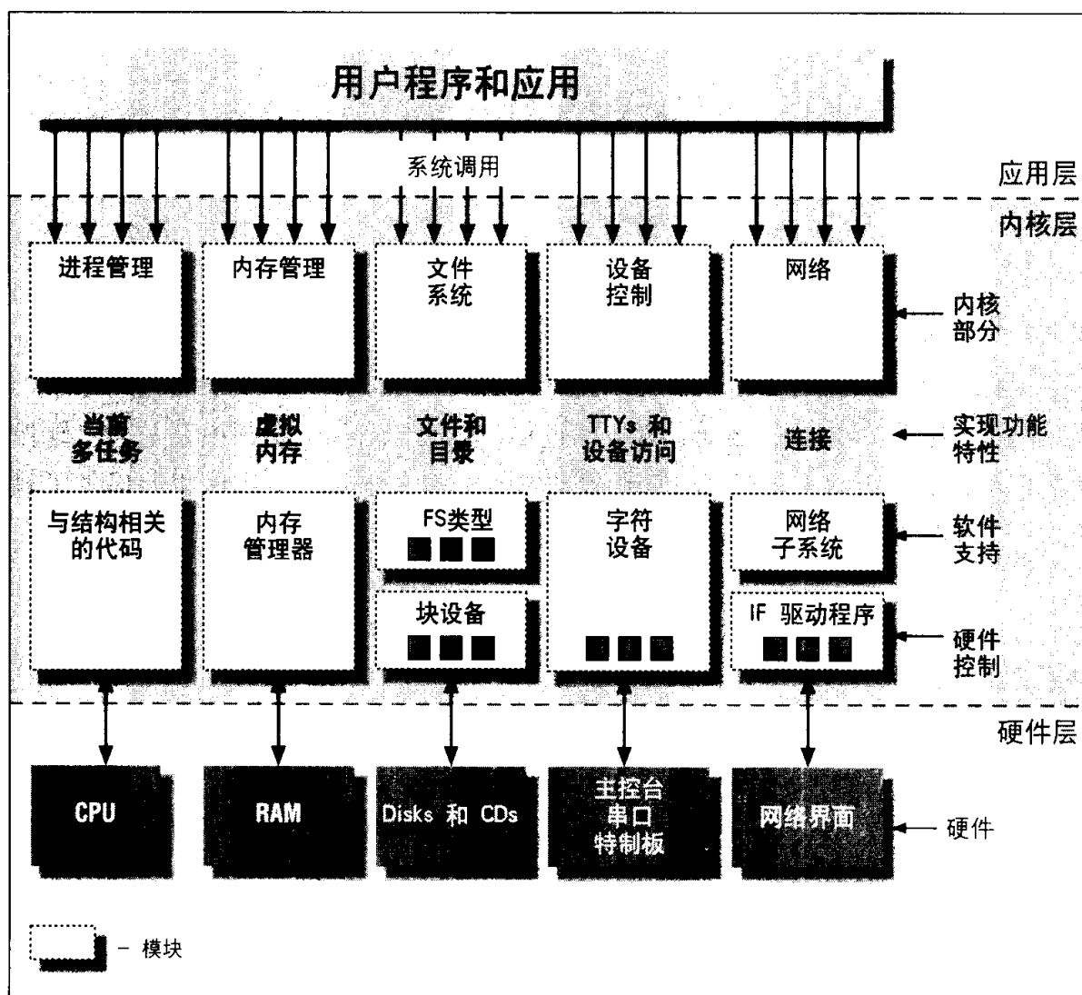
图 1-1 内核划分视图
