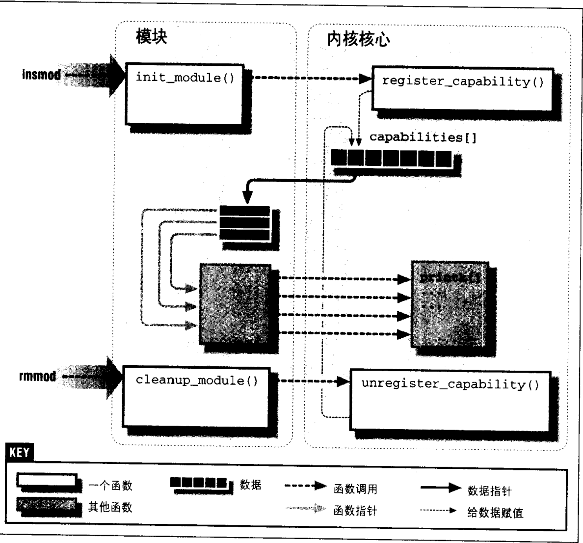
图 2-1 将一个模块连接到内核
