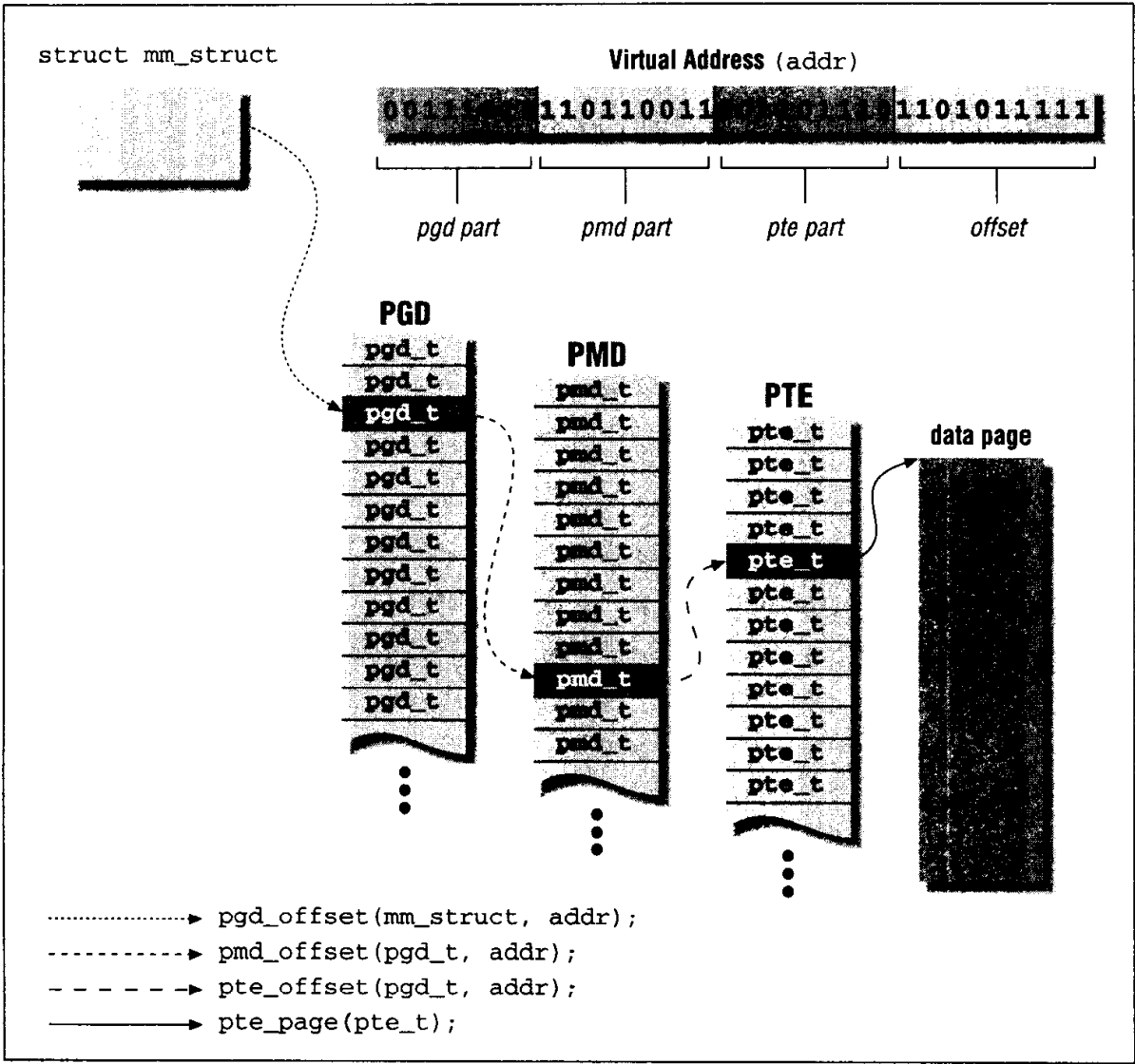
图 13-1 Linux 的三级页表
