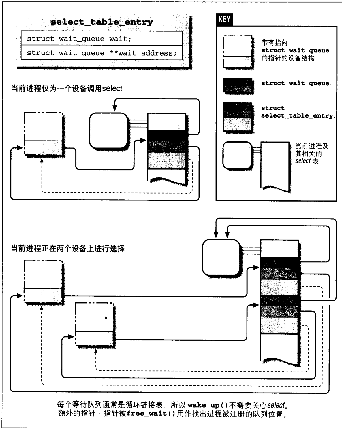
图 5-2 调用 select 的内部结构
