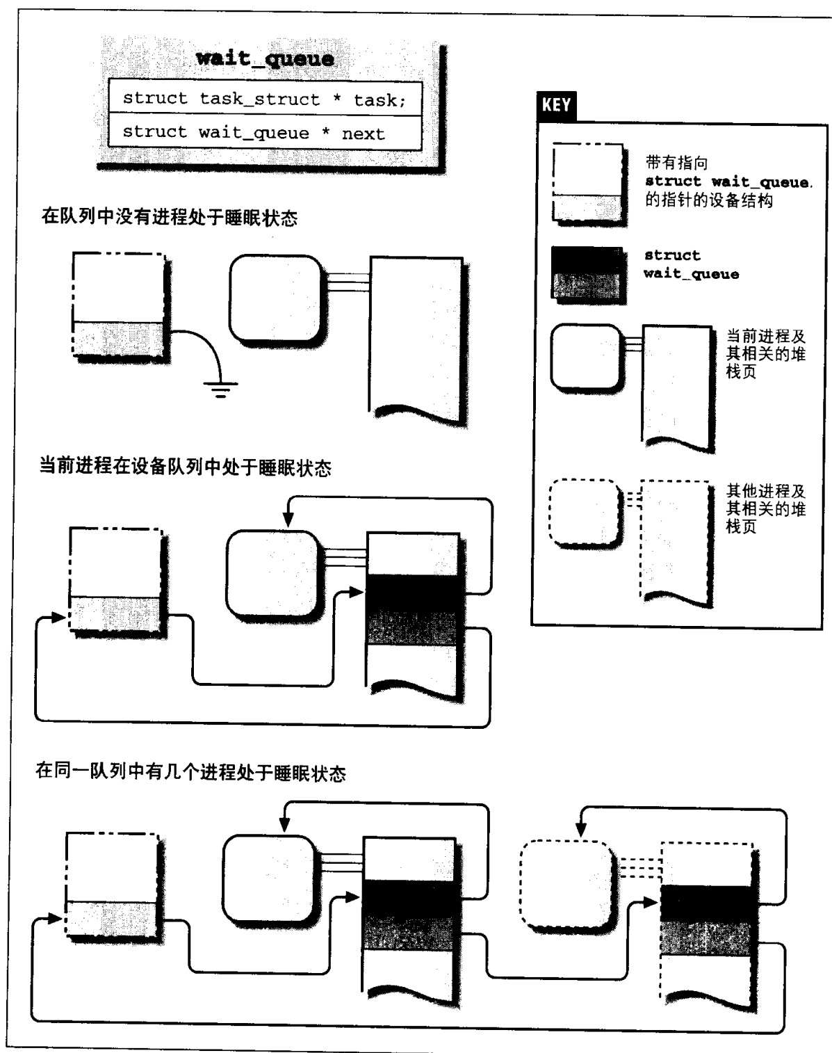
图 5-1 等待队列的工作示意
