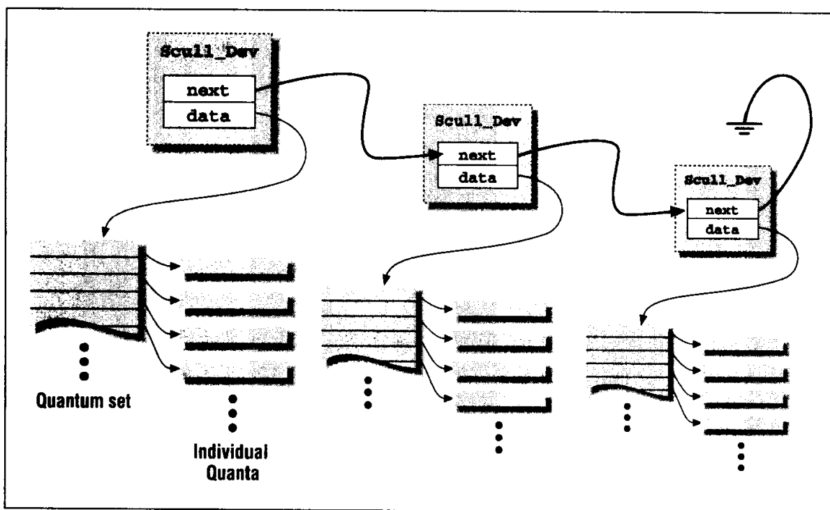
图 3-1 scull 设备的结构布局
