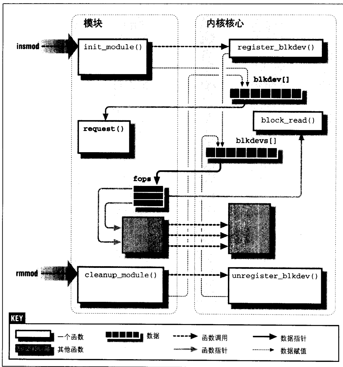
图 12-1 注册一个块设备驱动程序
