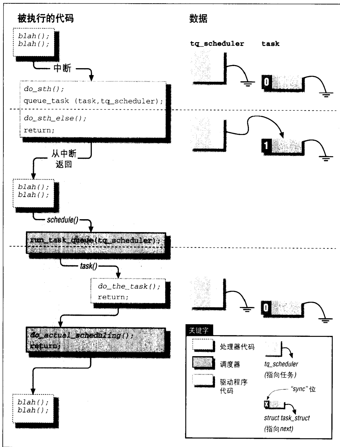
图 6-1 任务队列使用的执行流程
