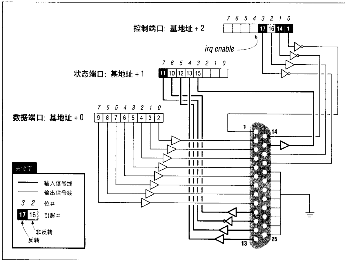
图 8-1 并口的插脚引线
