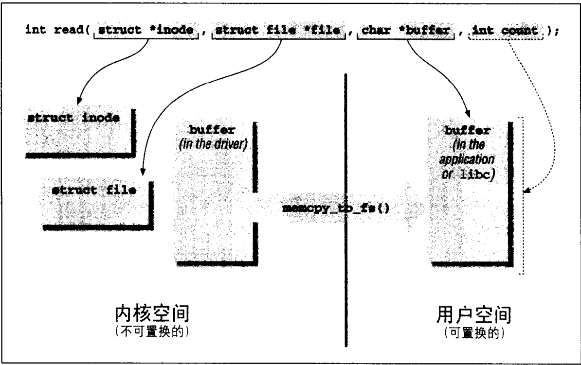
图 3-2 read 的参数
