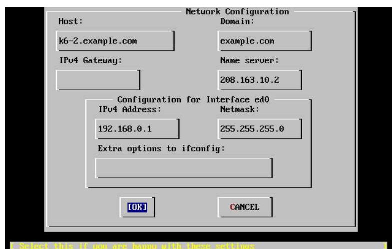
图2-32. 配置ed0接口
