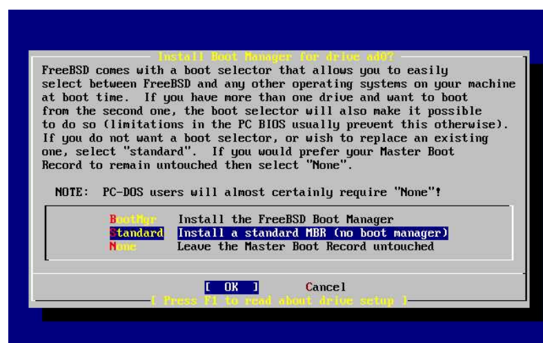
图2-19. Sysinstall 多重引导管理程序
