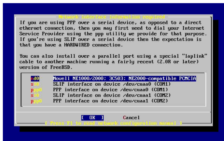
图2-31. 选择网卡设备
