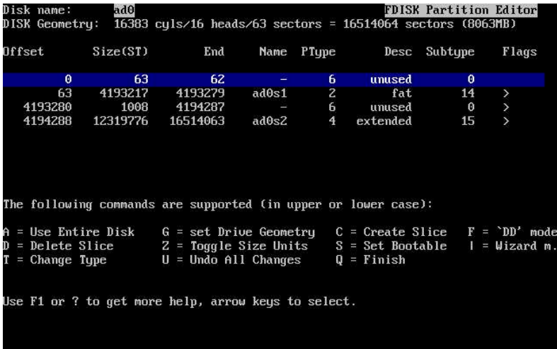
图2-17. 典型的尚未编辑前的Fdisk 分区表
