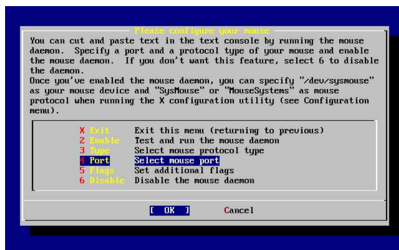
图2-47. 配置鼠标端口
