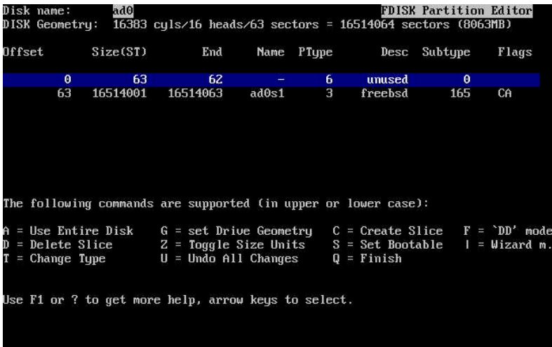
图2-18. Fdisk 分区使用整个硬盘
