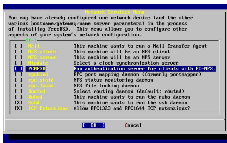
图2-54. 网络配置之下层配置
