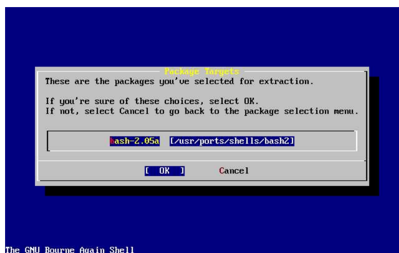
图2-60. 确认安装的软件包
