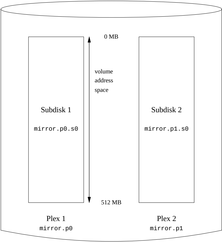
图19-5. 镜像Vinum 卷
