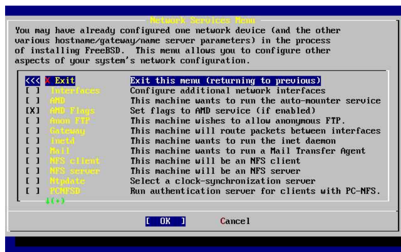
图2-51. 网络配置之上层配置
