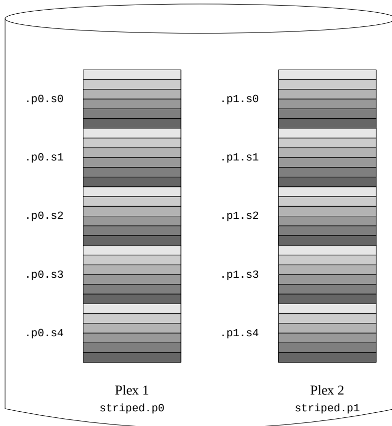
图19-7. 镜像并条带化的Vinum 卷
