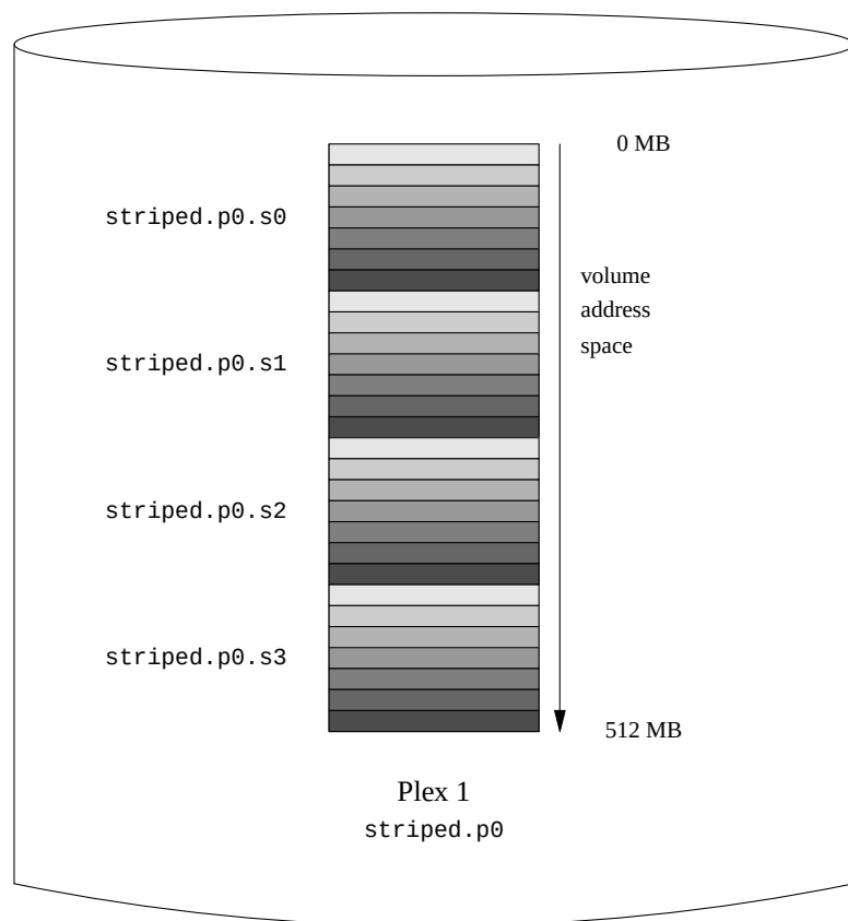
图19-6. 条带化的Vinum 卷
