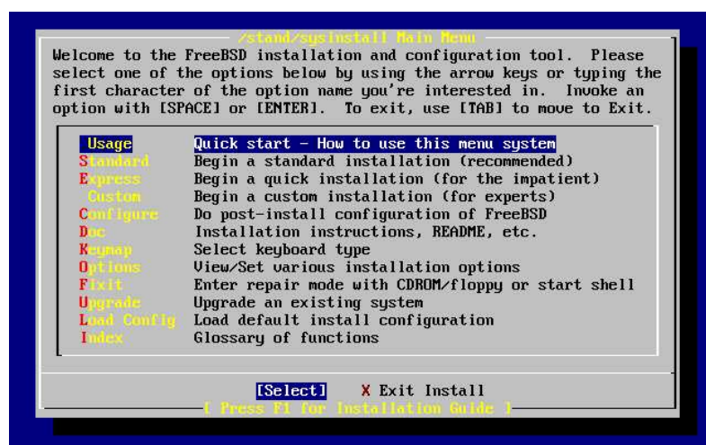
图2-8. 选取Sysinstall 主菜单的Usage 项目
