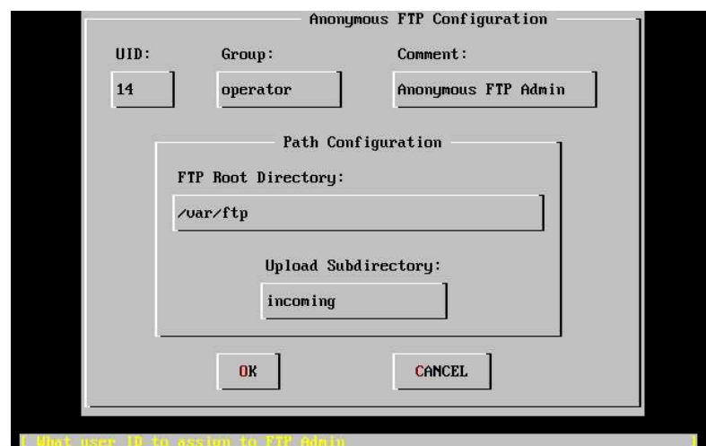
图2-34. 默认的匿名FTP 配置
