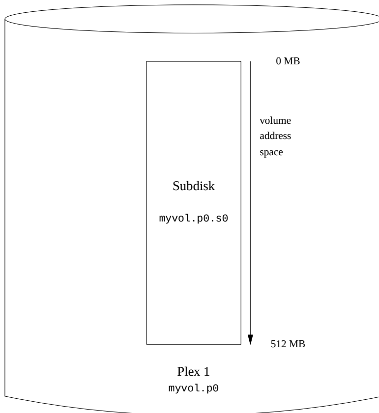
图19-4. 一个简单的Vinum 卷
