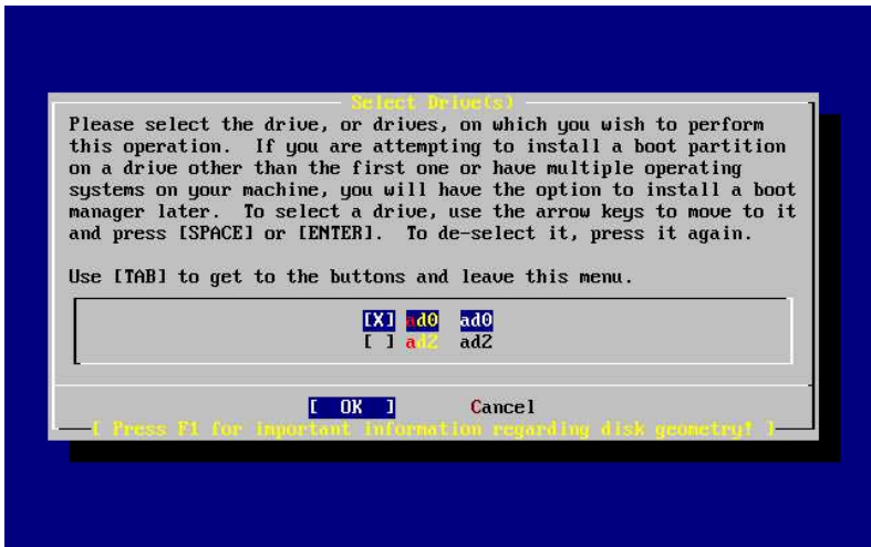
图2-20. 离开选择硬盘画面
