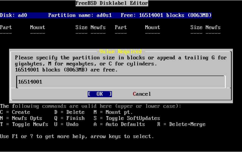
图2-23. 根目录使用空间
