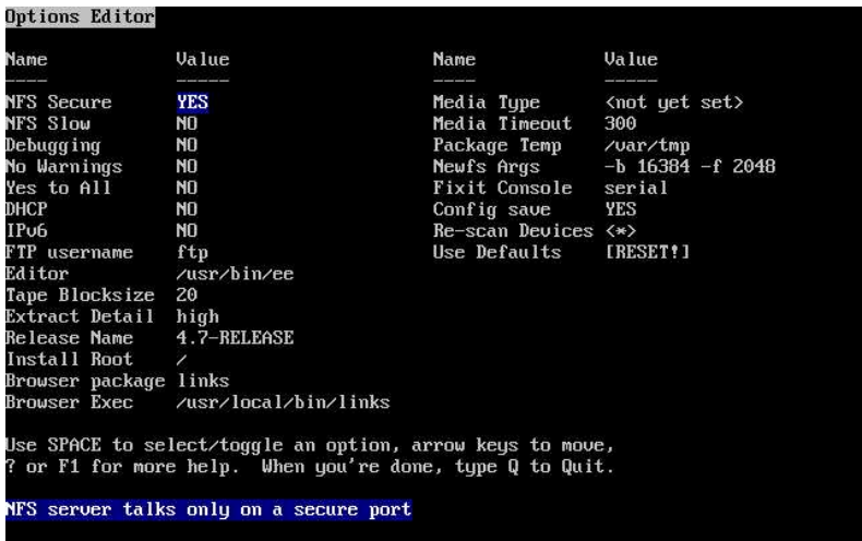
图2-14. Sysinstall 选项设置
