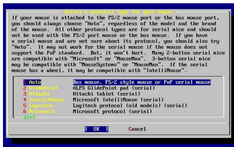
图2-46. 设置鼠标协议
