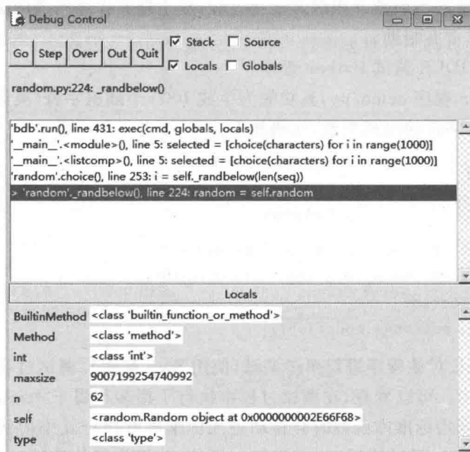
图 7-4 程序调试截图(二)
