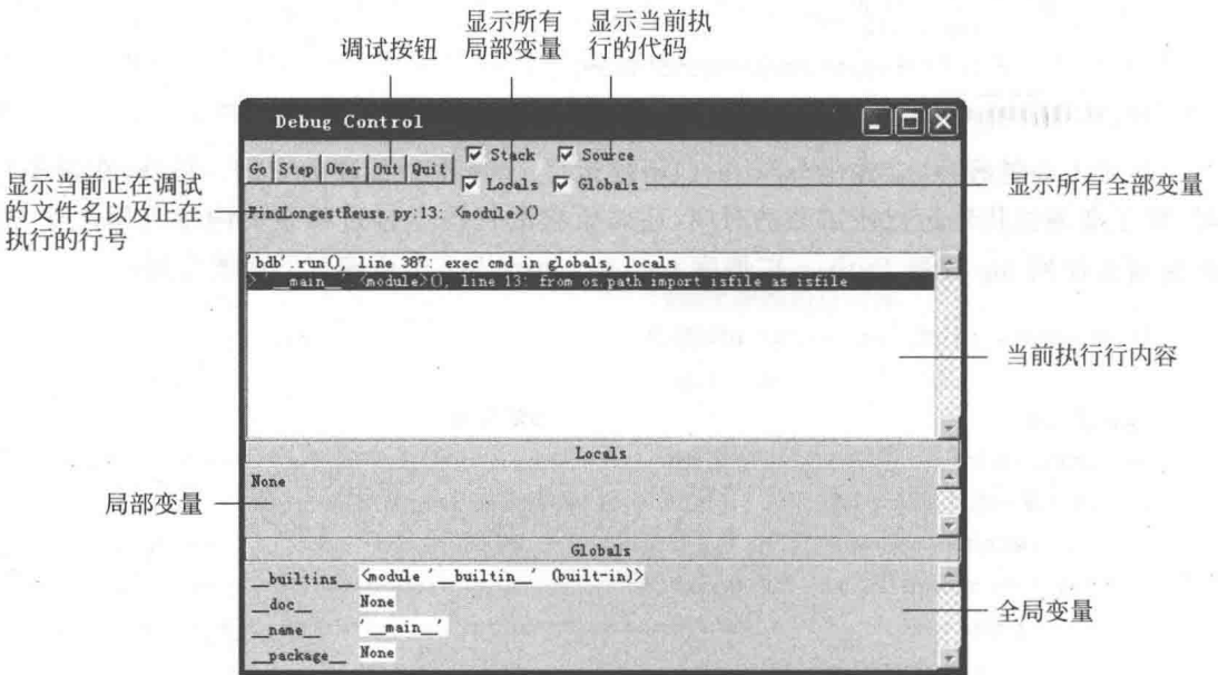
图 7-2 IDLE 调试器窗口
