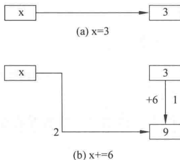
图 1-11 Python 内存管理模式
