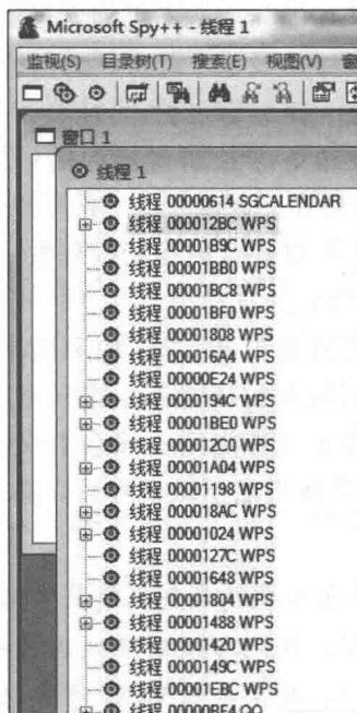
图 10-4 WPS 创建的部分线程
