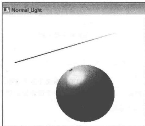
图 12-3 光照模型
