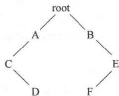
图 4-3 二叉树
