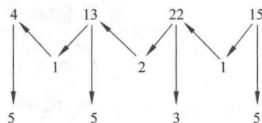
图 3-9 把卷积结果转换为数字
