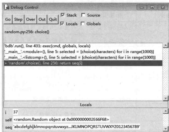
图 7-6 程序调试截图(四)
