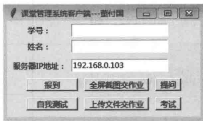
图 16-2 学生端主界面
