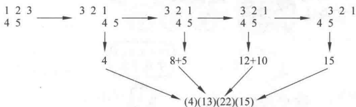
图 3-8 一维序列卷积计算原理示意图
