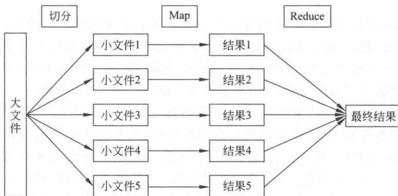
图 11-1 MapReduce 流程
