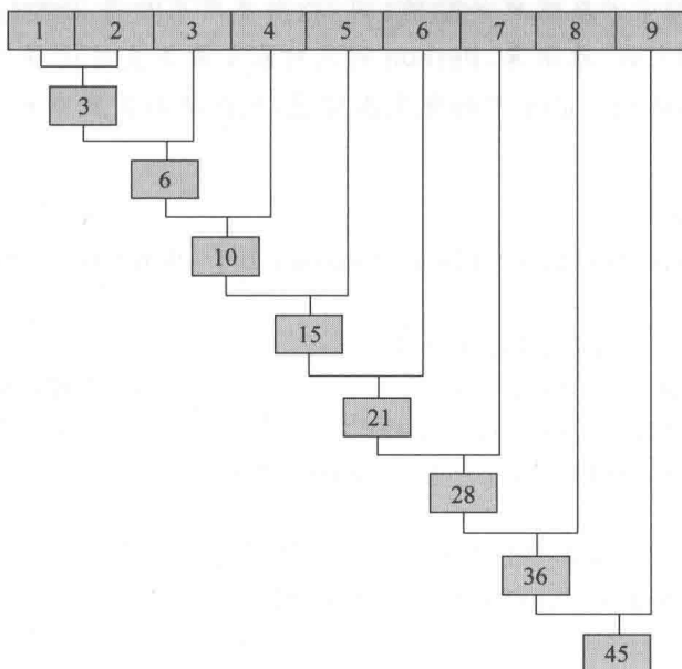
图 2-3 reduce()函数执行过程示意图
