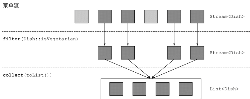
图 5-1 用谓词筛选一个流
