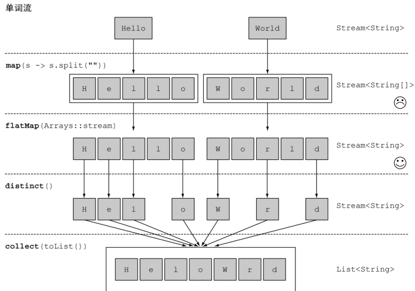
图 5-6 使用flatMap找出单词列表中各不相同的字符
