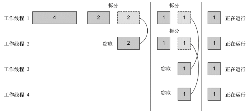
图 7-5 分支/合并框架使用的工作窃取算法
