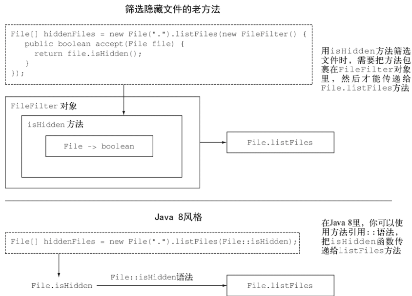
图 1-4 将方法引用 File::isHidden 传递给 listFiles 方法
