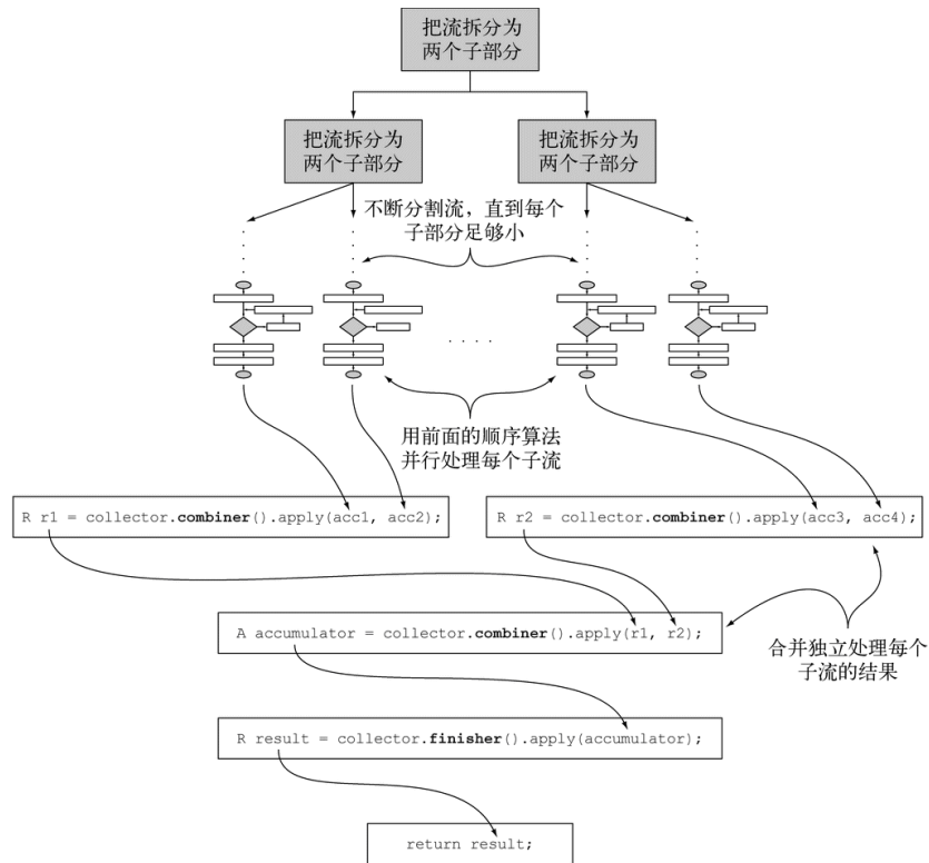
图 6-8 使用combiner方法来并行化归约过程
