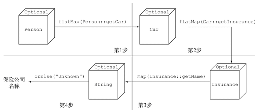
图 10-5 使用Optional解引用串接的Person/Car/Insurance
