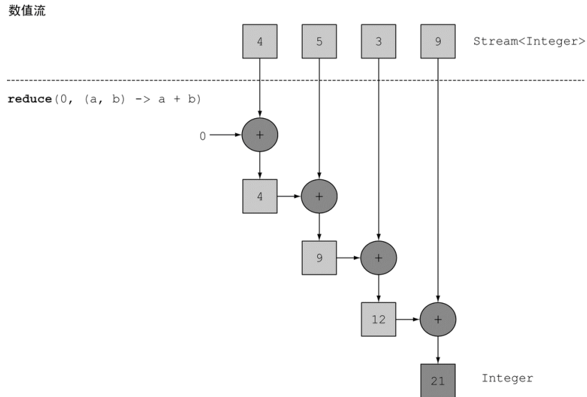
图 5-7 使用reduce来对流中的数字求和
