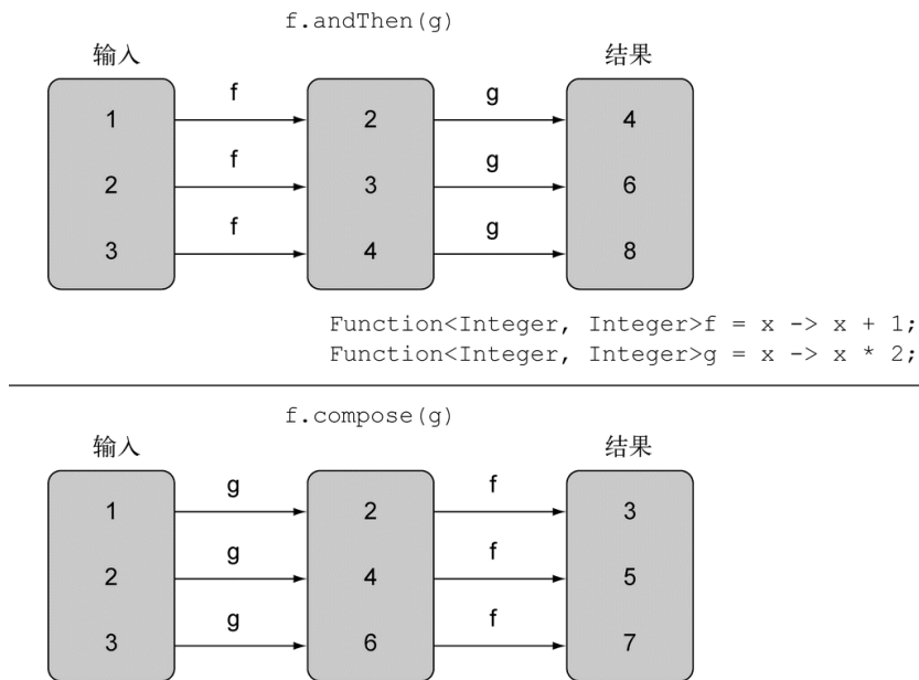
图 3-6 使用 andThen 与 compose
