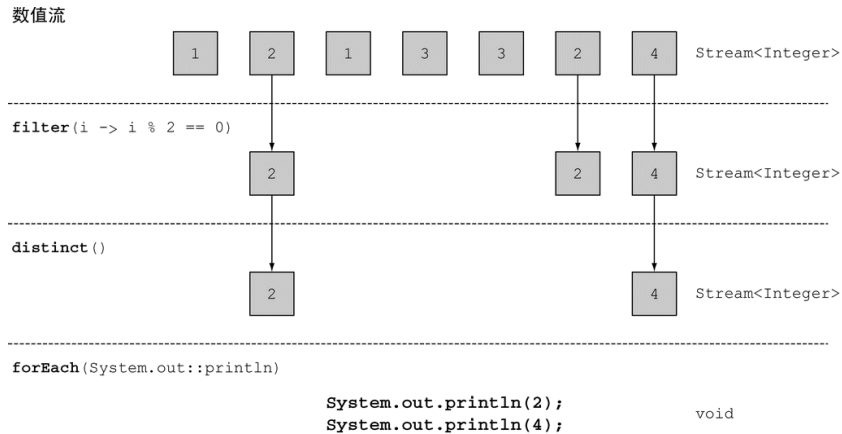
图 5-2 筛选流中各异元素
