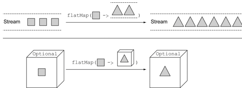
图 10-4 Stream 和 Optional 的 flatMap 方法对比
