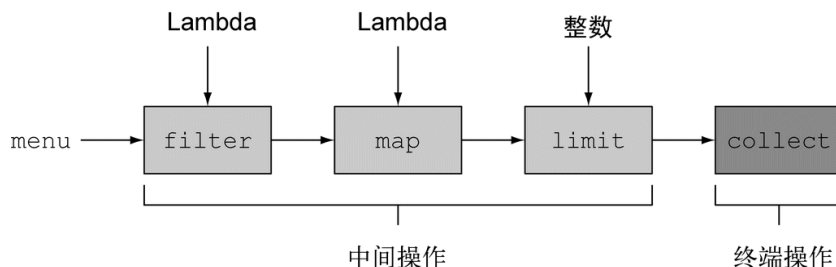
图 4-5 中间操作与终端操作
