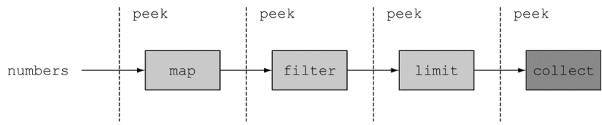
图 8-4 使用peek查看Stream流水线中的数据流的值
