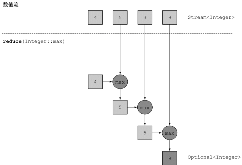
图 5-8 一个归约操作——计算最大值
