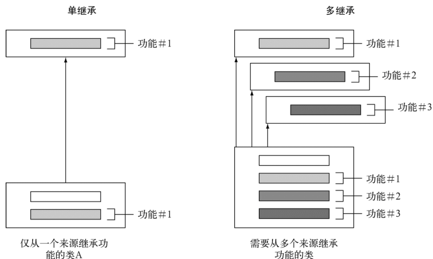
图 9-3 单继承和多继承的比较
