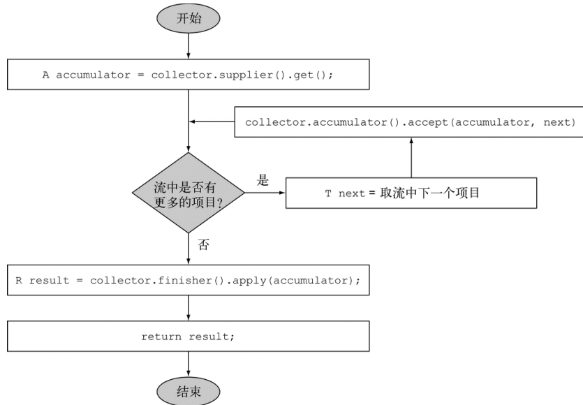
图 6-7 顺序归约过程的逻辑步骤
