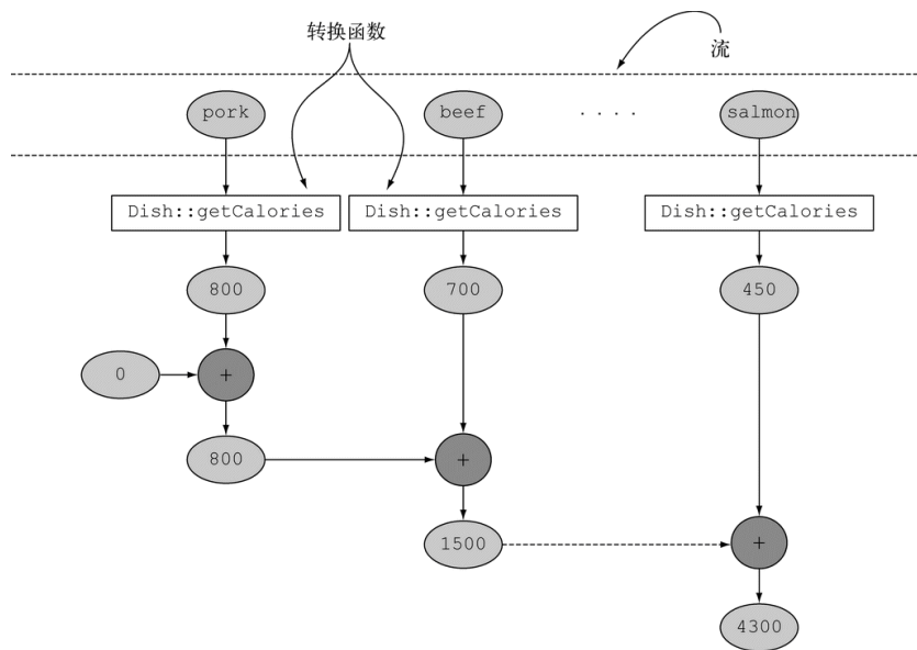
图 6-2 summingInt 收集器的累积过程
