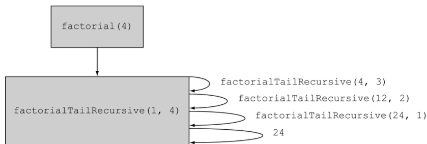
图 13-6 阶乘的尾-递归定义，这里它只使用了一个栈帧
