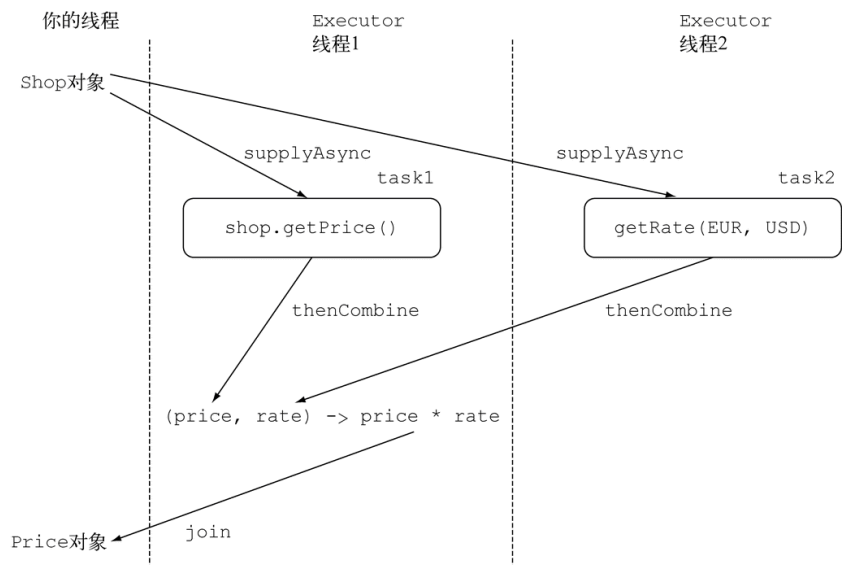
图 11-6 合并两个相互独立的异步任务
