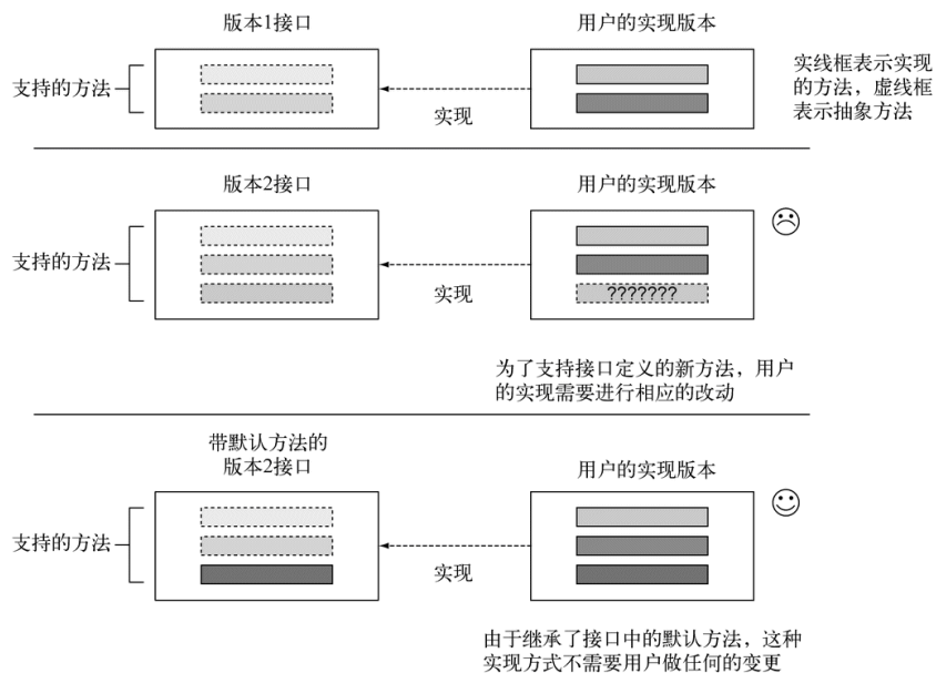
图 9-1 向接口添加方法
