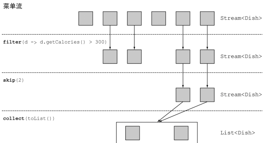
图 5-4 在流中跳过元素
