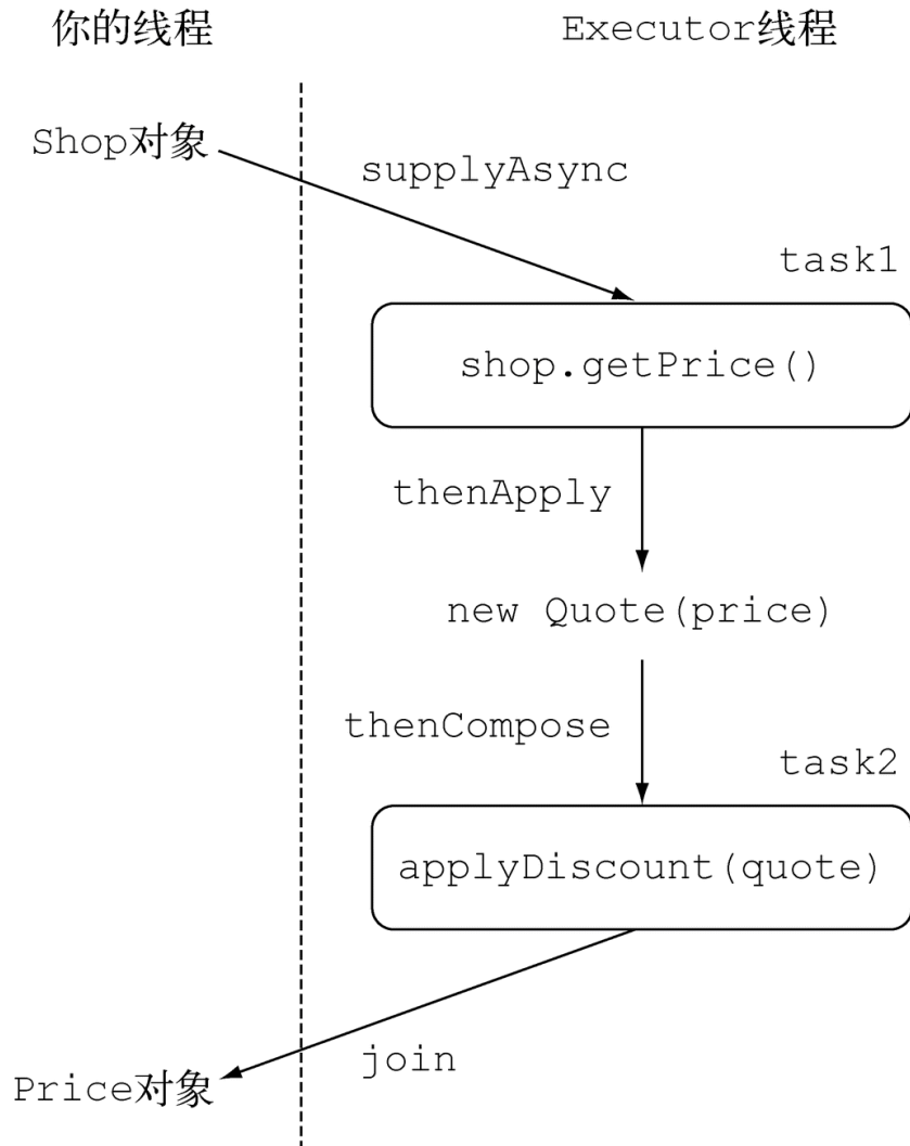
图 11-5 构造同步操作和异步任务
