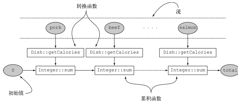
图 6-3 计算菜单总热量的归约过程
