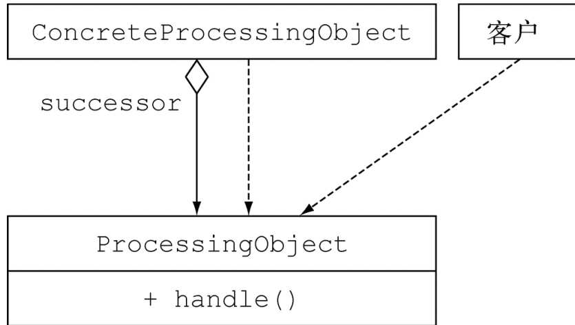
图 8-3 责任链设计模式
