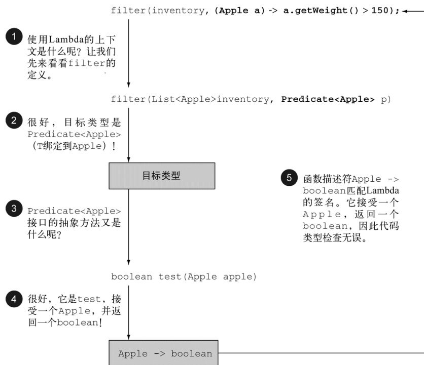
图 3-4 解读Lambda表达式的类型检查过程
