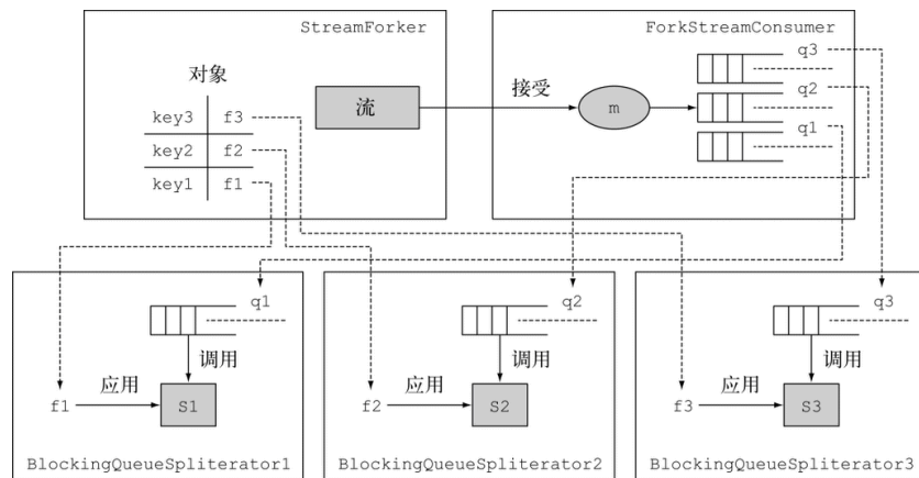
图 C-2 StreamForker及其合作的构造块
