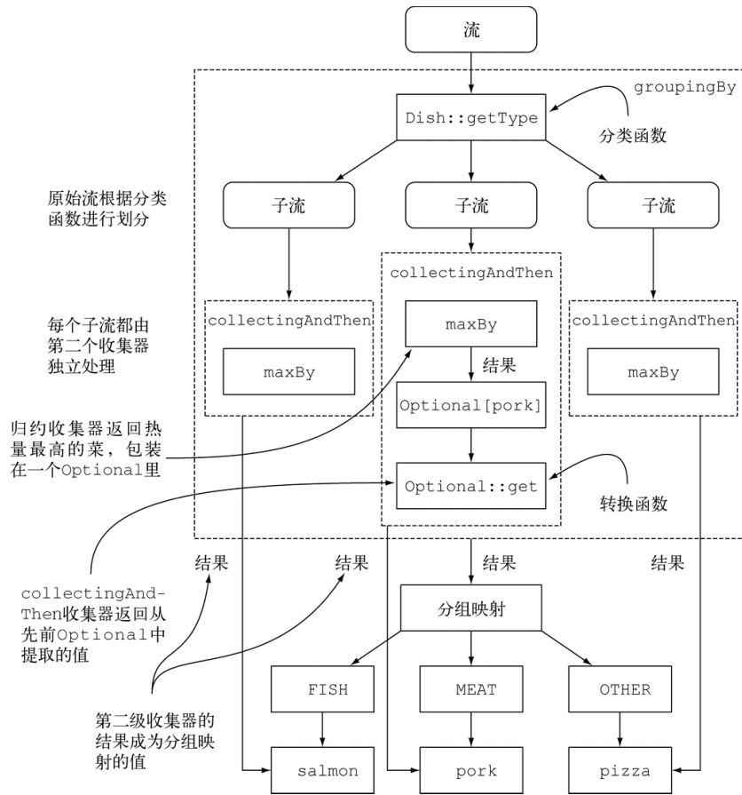
图 6-6 嵌套收集器来获得多重效果
