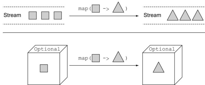
图 10-2 Stream和Optional的map方法对比
