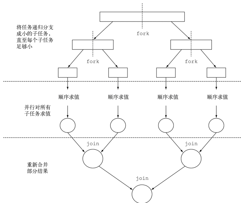
图 7-3 分支/合并过程
