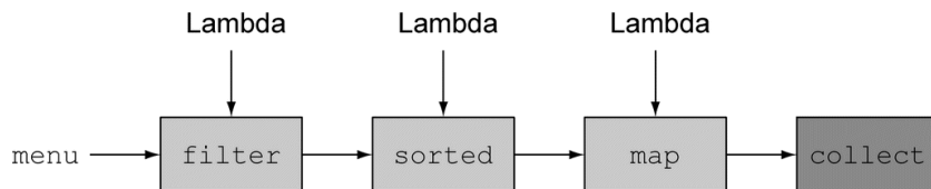
图 4-1 将流操作链接起来构成流的流水线
