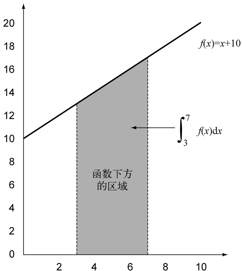
图 3-8 函数 f(x)=x+10 ， x 从3到7下方的面积
