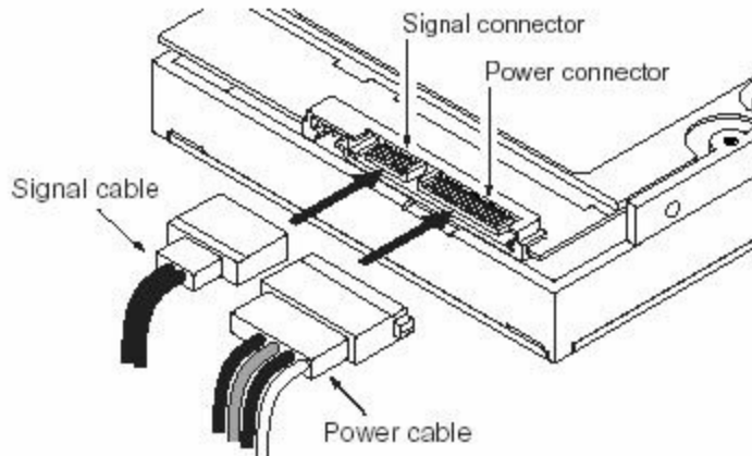
图0.2.6、SATA 接口的排线（图示取自 Seagate 网站）
