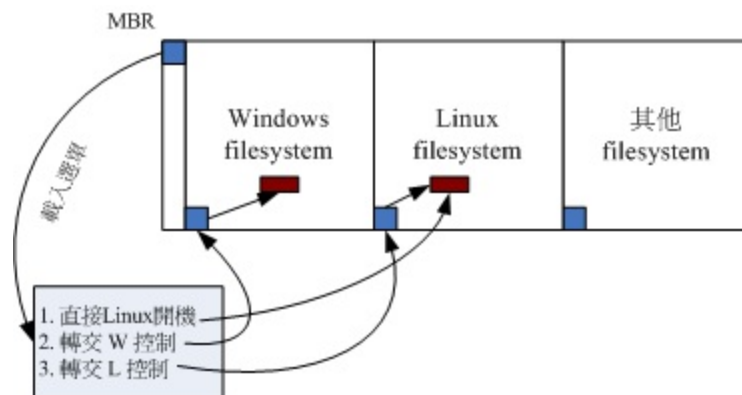
图19.1.2、开机管理程序的菜单功能与控制权转交功能示意图
