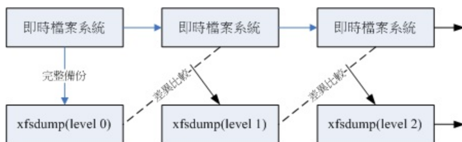
图8.4.1、xfsdump 运行时，完整备份与累积备份示意图
