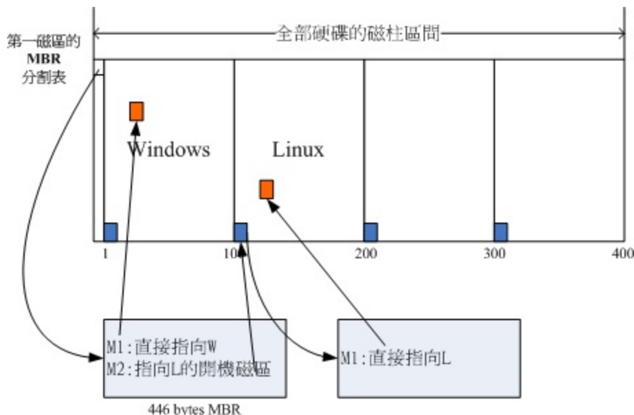
图2.2.8、开机管理程序的工作执行示意图
