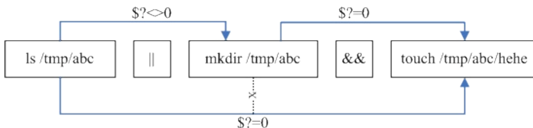
图10.5.2、指令依序执行的关系示意图
