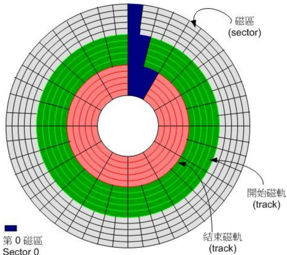
图2.2.1、盘片组成示意图
