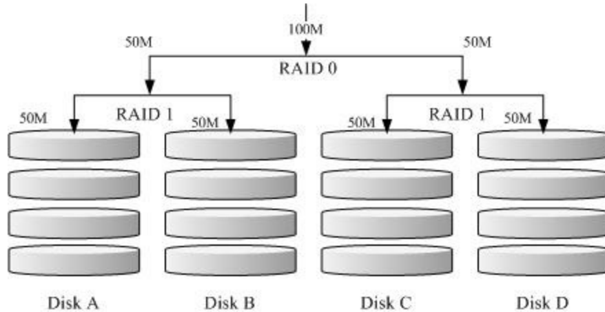
图14.2.3、RAID-1+0 的磁盘写入示意图
