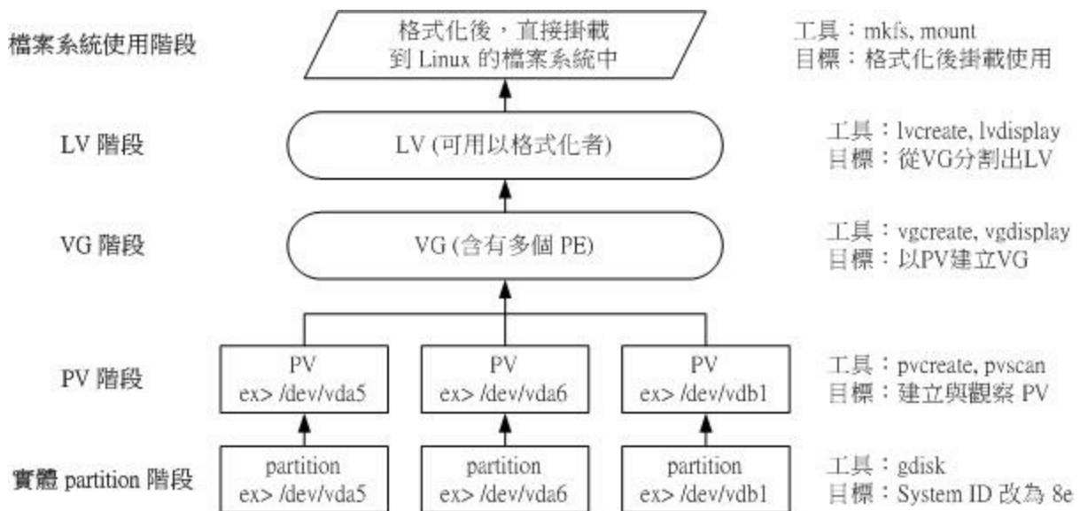
图14.3.2、LVM 各元件的实现流程图示
