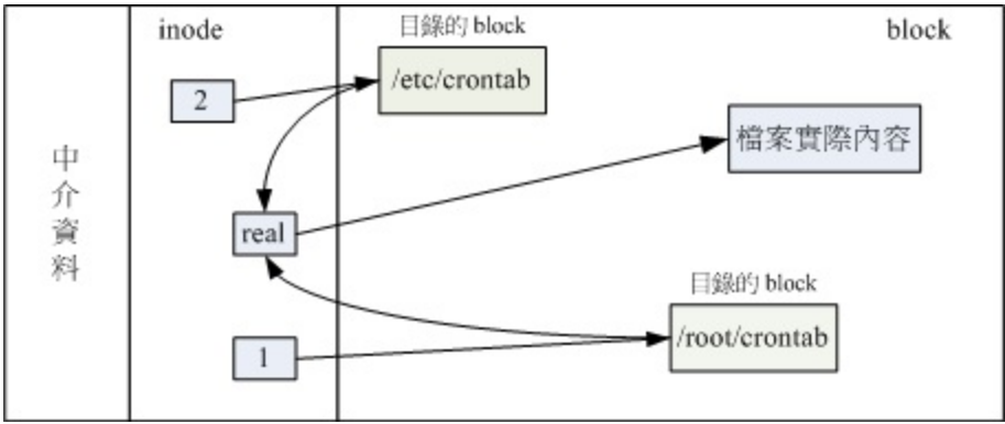
图7.2.1、实体链接的文件读取示意图
