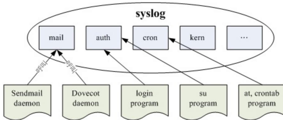
图18.2.1、syslog 所制订的服务名称与软件调用的方式
