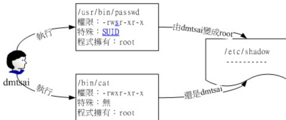
图6.4.1、SUID程序执行的过程示意图
