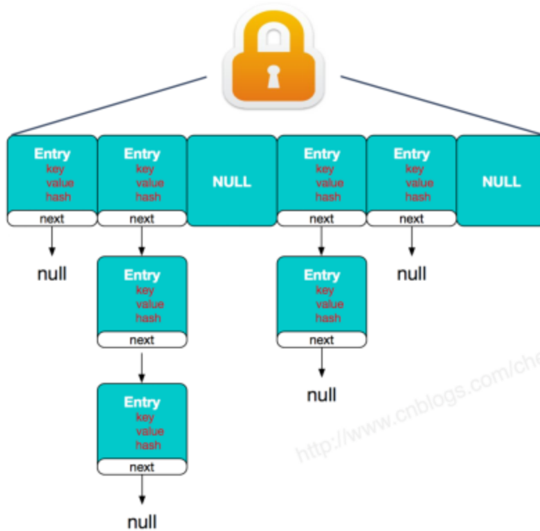
HashTable 全表锁
