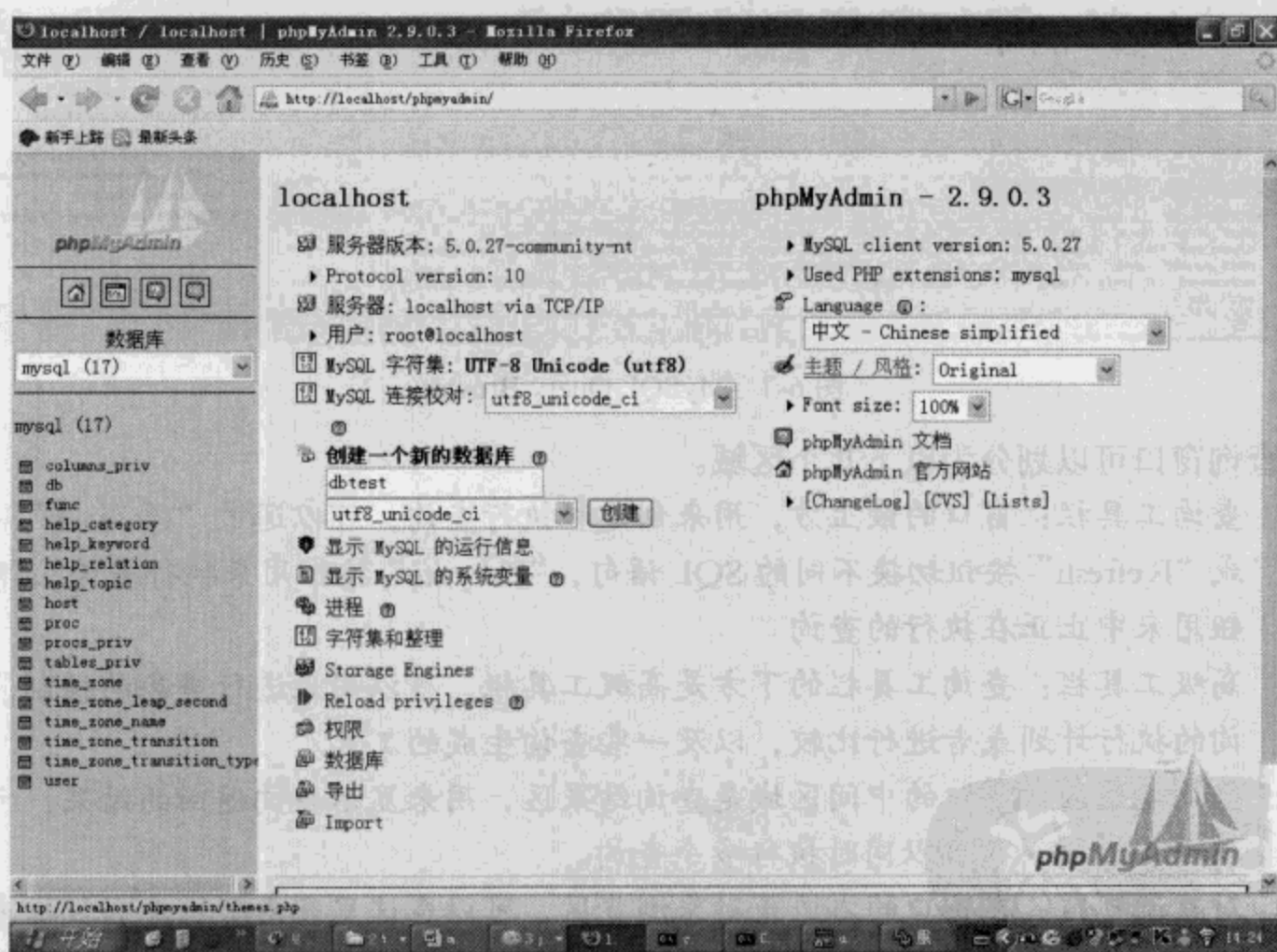
图 6-8 phpMyAdmin 主页面
