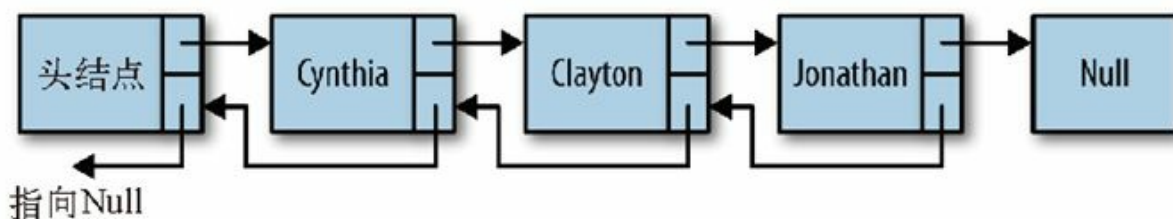
图6-5：双向链表
