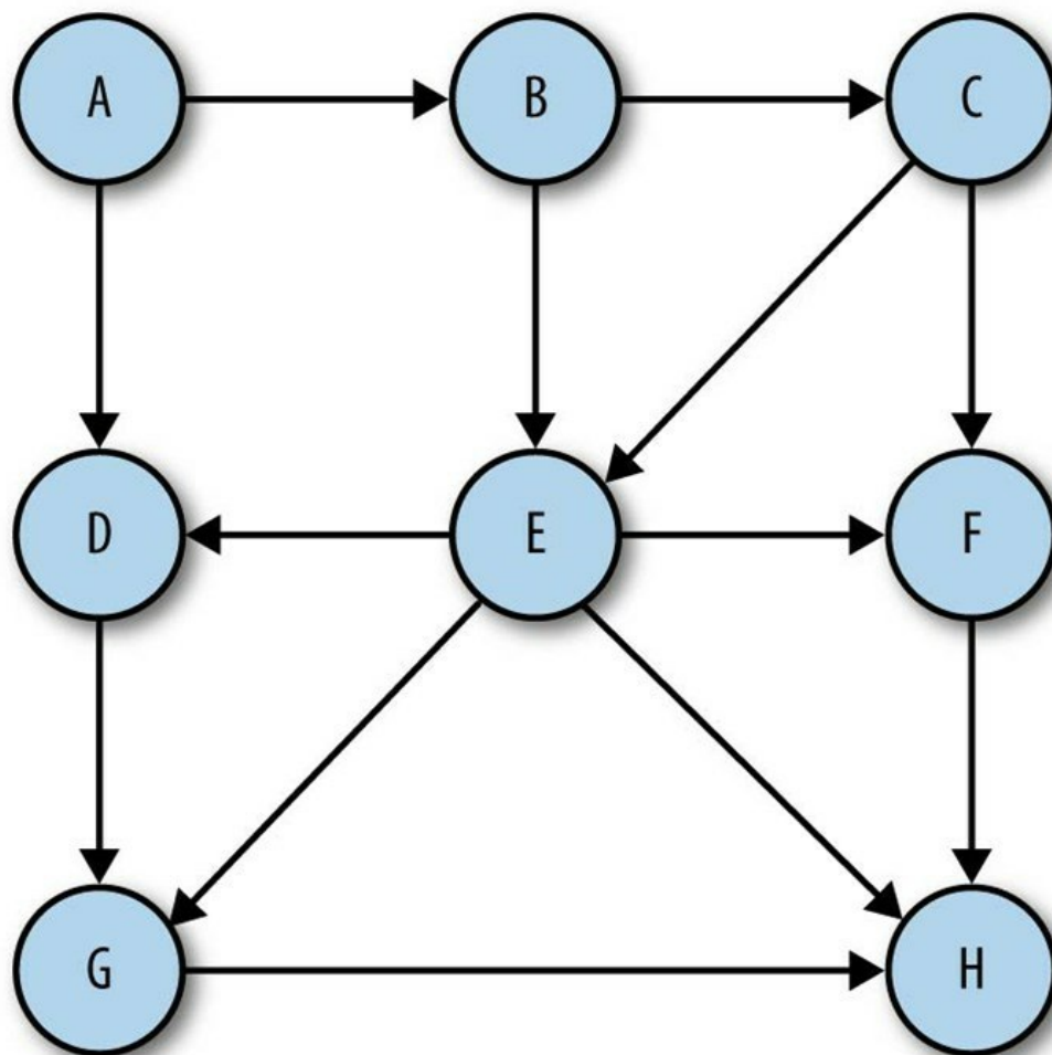
图11-1：有向图
